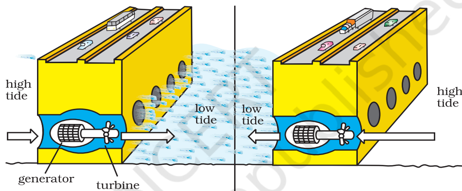
Fig. 3.22: Tidal Energy
